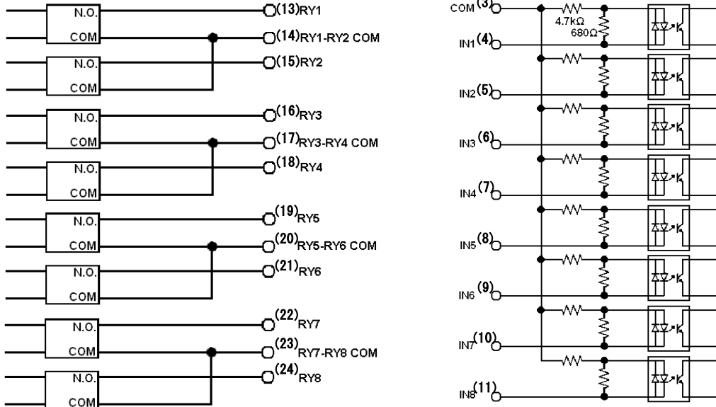
端子台接続図
