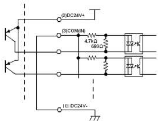
PNP 接続
