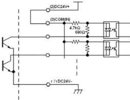
NPN 接続
